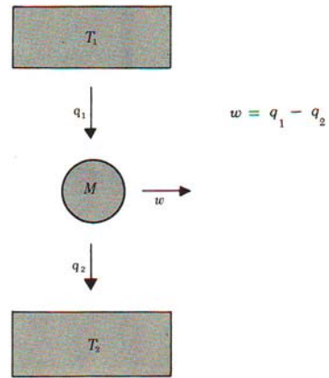
Fig. 5.11.4 A real engine
