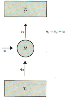
Fig. 5·12·1 A real refrigerator.
